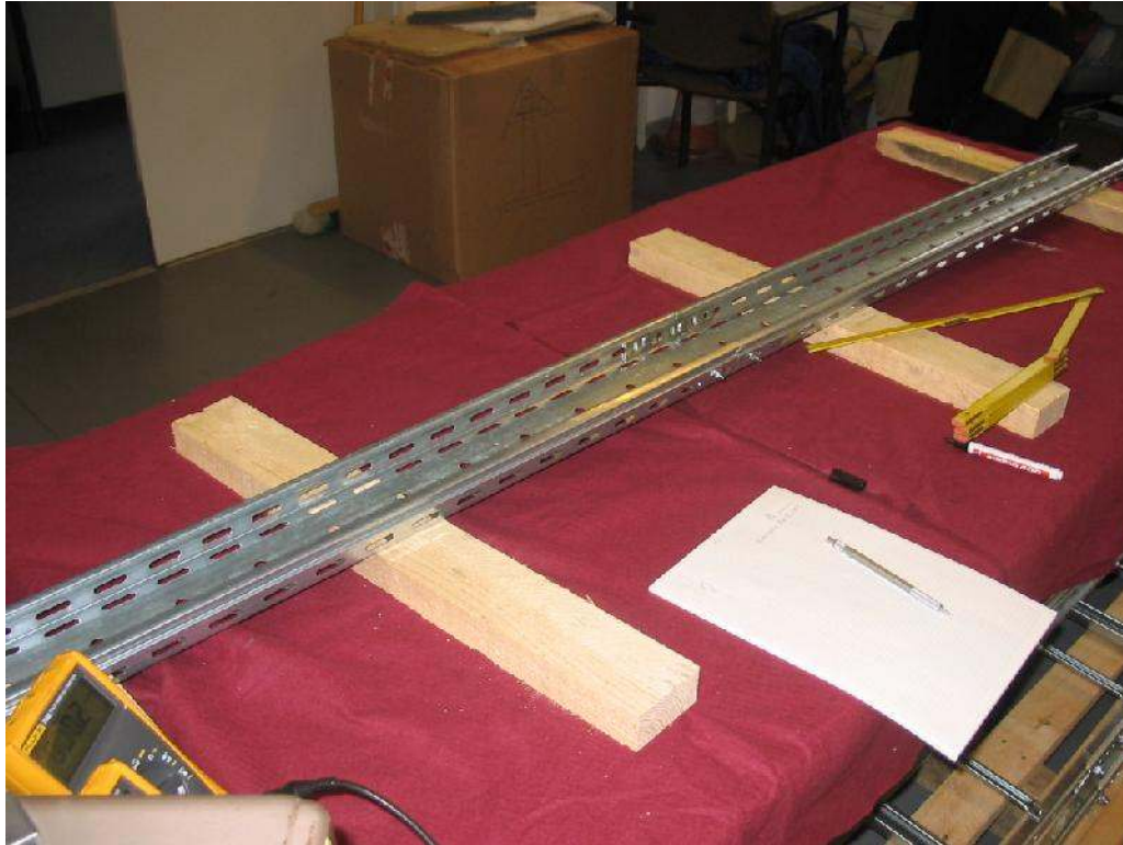
Bild / Picture 6: Kabelrinne RI 60-05 S
