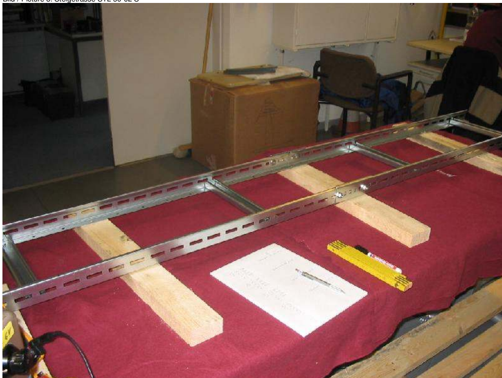
Bild / Picture 8: Steigtrasse STL 50-02 S
